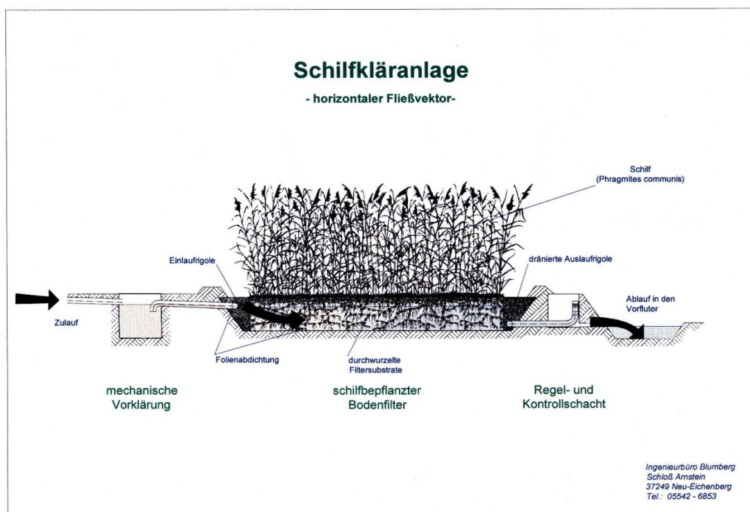
(Schemaskizze zum Schilfklärverfahren, Variante mit horizontalem Fließvektor)
